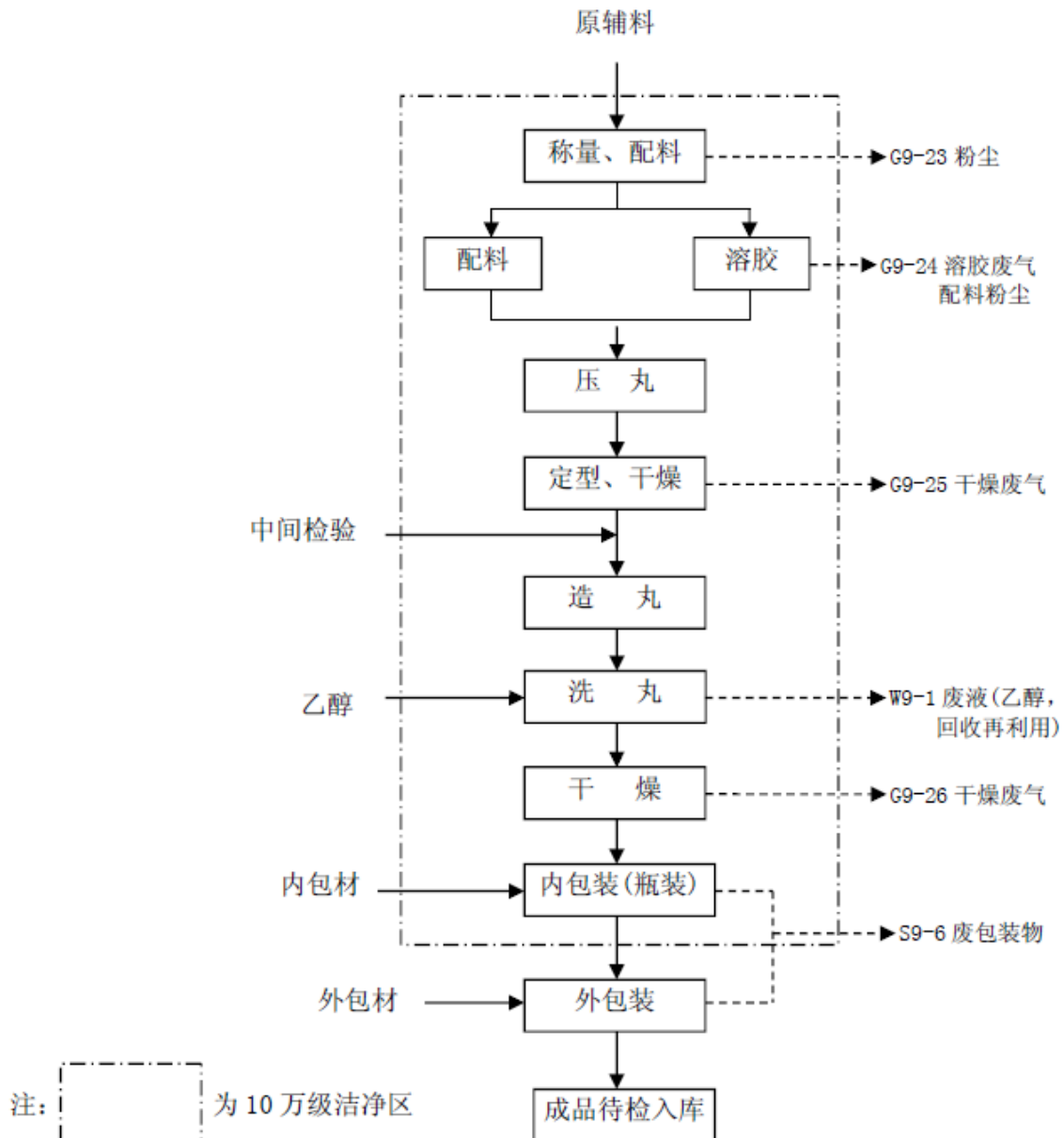
图 2-17 软胶囊生产线生产工艺流程图
