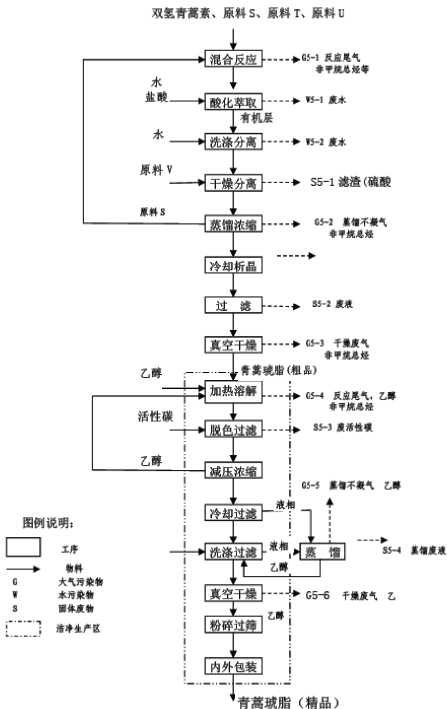
图 2-6 青蒿琥脂生产工艺及产污环节图
