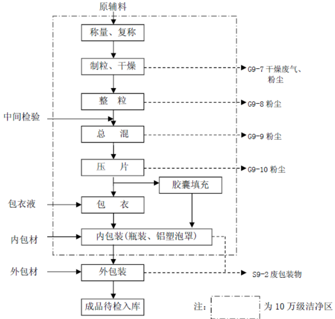
图 2-13 白品种（片剂、胶囊剂）生产工艺流程图
