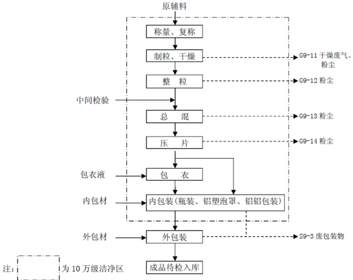
图 2-14 黄品种片剂生产工艺流程图
