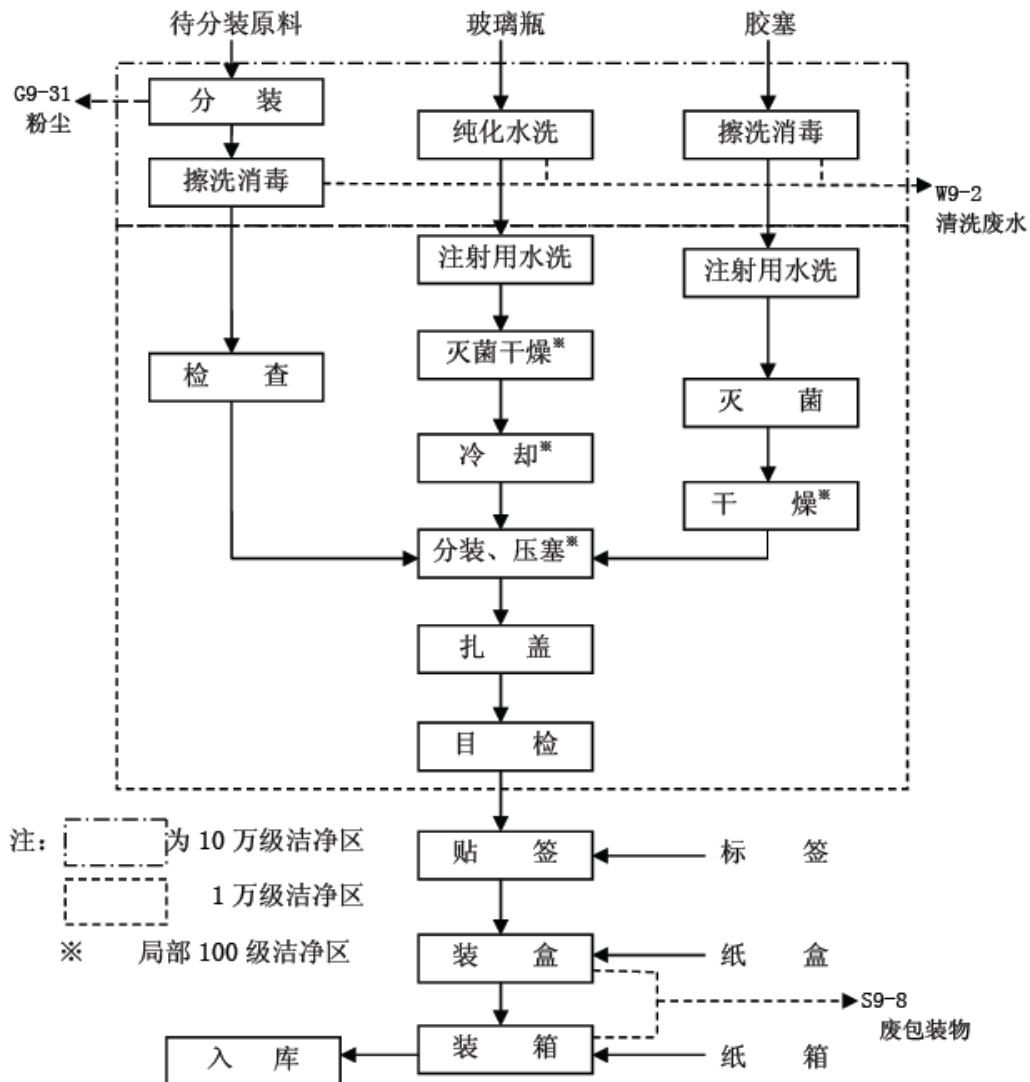
图 2-19 针剂生产工艺流程图
