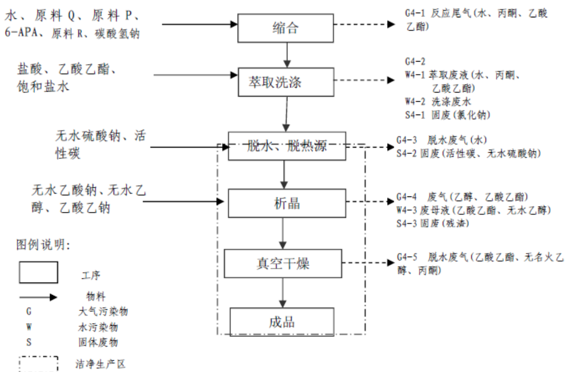
图 2-5 氟氯西林钠生产工艺及产污环节图
