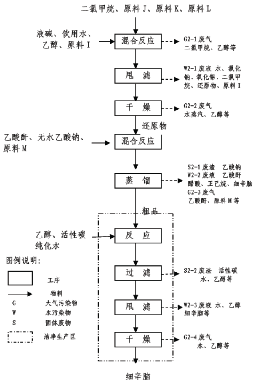
图 2-3 细辛脑生产工艺及产污环节图
