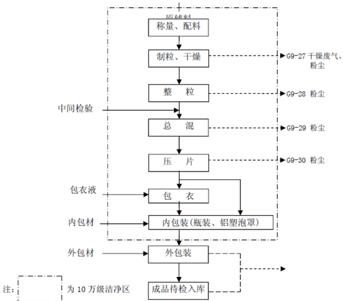
图 2-18 OEM 固体制剂生产工艺流程图
