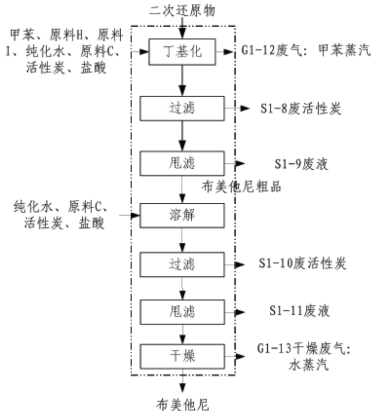
图 2-2 布美他尼生产工艺流程图
