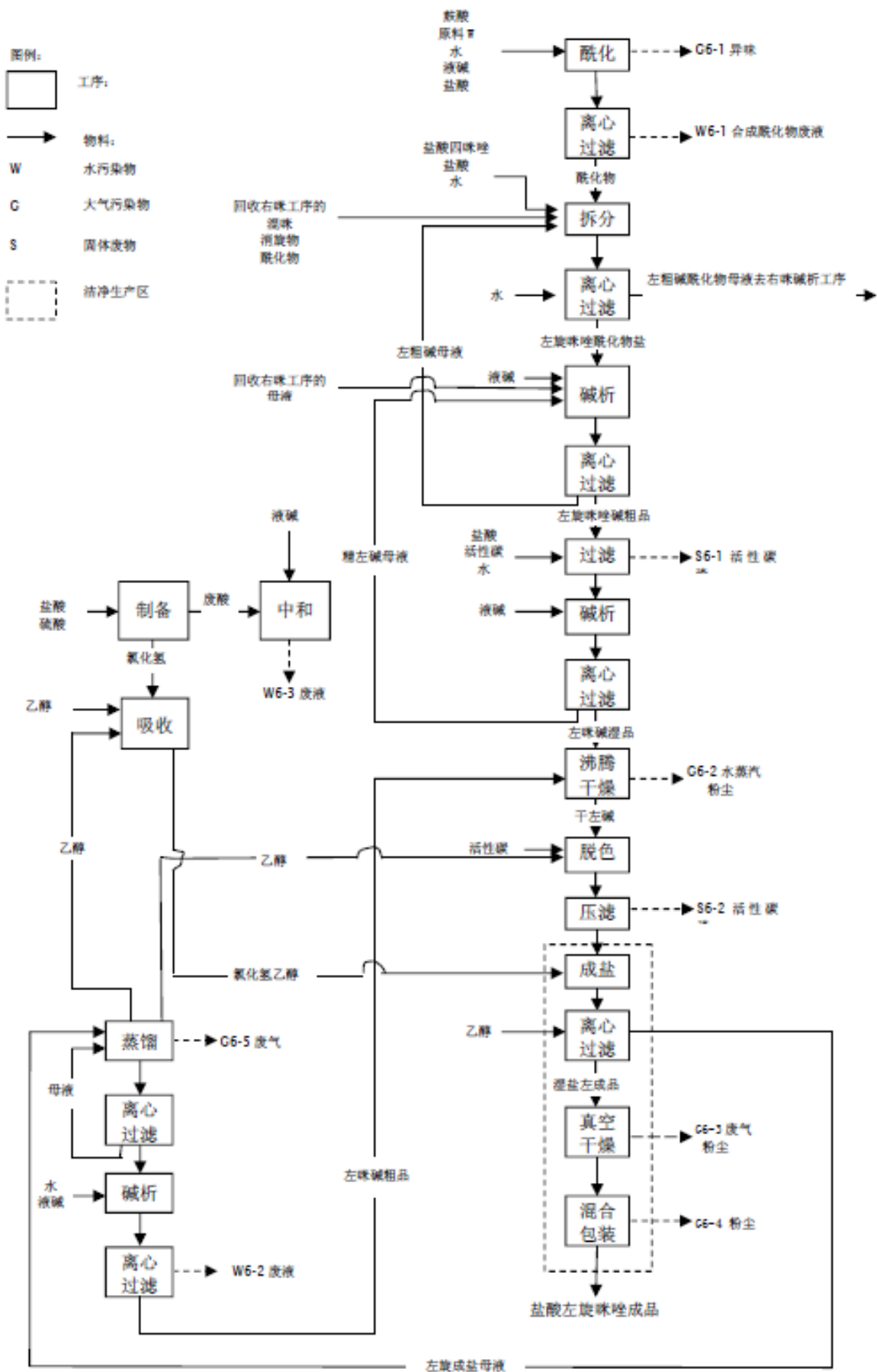
图 2-8 盐酸左旋咪唑工艺流程图
