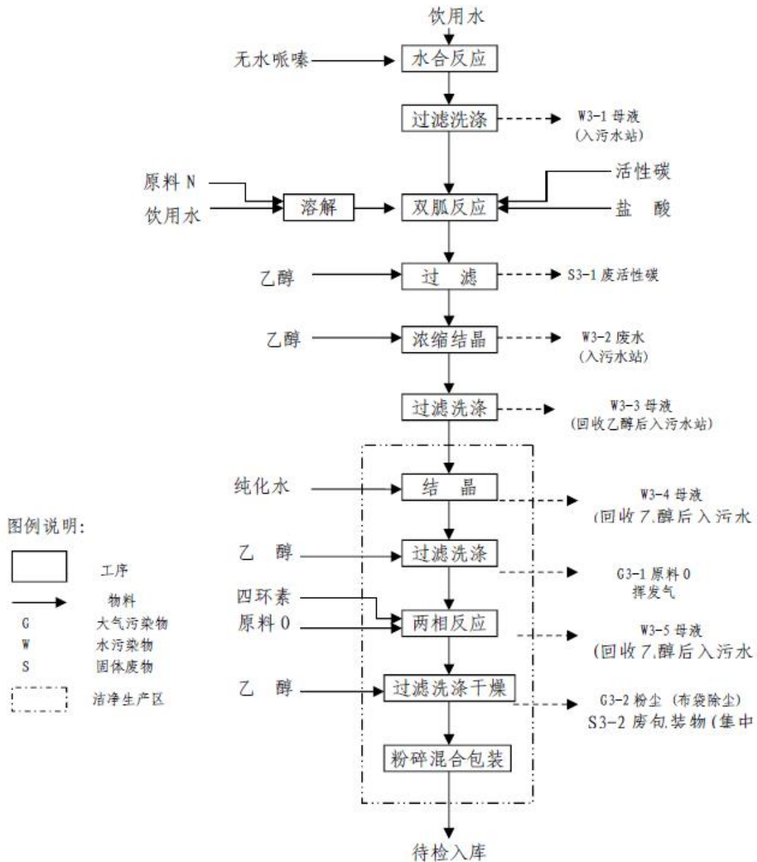
图 2-4 盐酸胍甲环素生产工艺及产污环节图
