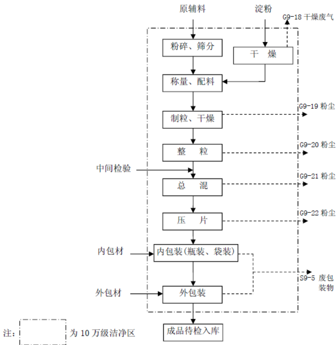
图 2-16 乳酶生制剂生产工艺流程图
