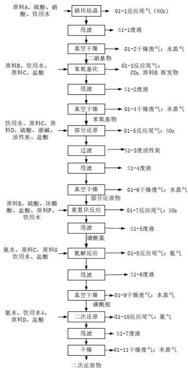
图 2-1 布美他尼生产工艺流程图
