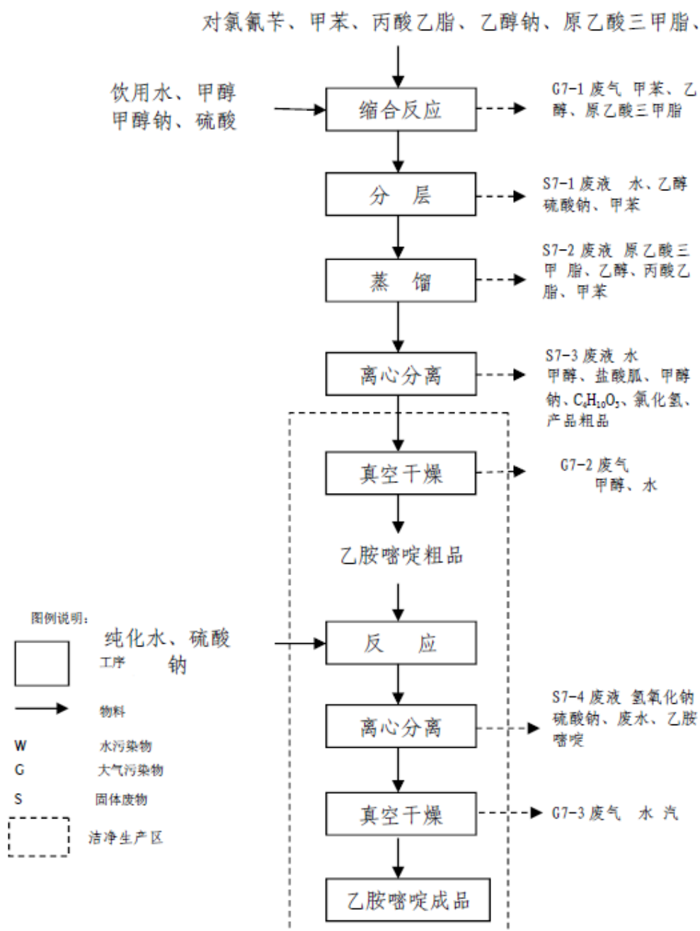
图 2-9 乙胺嘧啶工艺流程图
