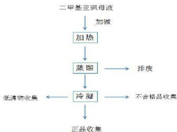
图 2-7 二甲基亚砷回收工艺流程图
